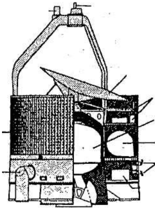
antenna discoidale a l'ingno raggio sensori scientifici motore del razzo carburante di spinta condotti di spinta * — sensori scientifici
